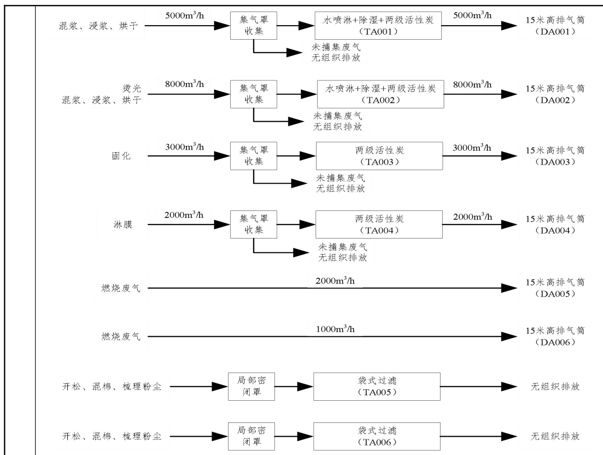
图 4-1 企业废气处理工艺图
