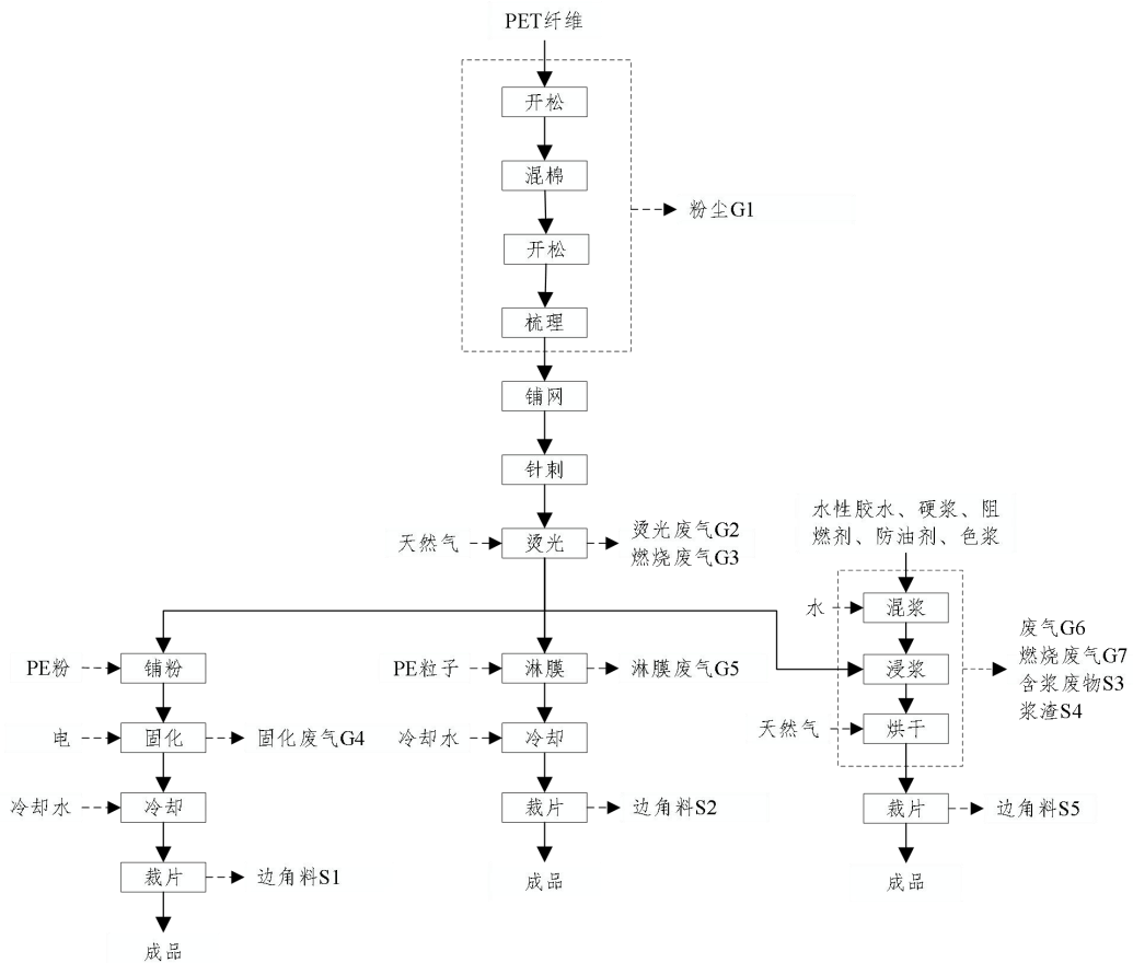
图 2-3 工艺流程图
