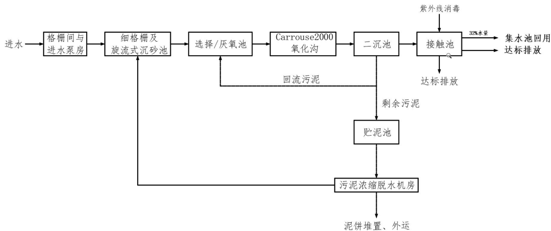
图 4-2 污水处理厂工艺图
