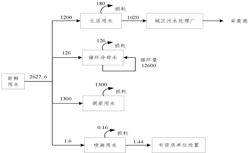
图 2-2 项目水平衡图 (t/a)
