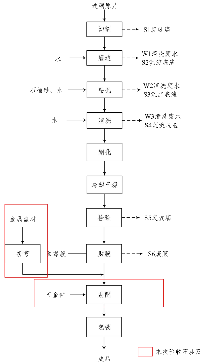
图 2-2 工艺流程图
