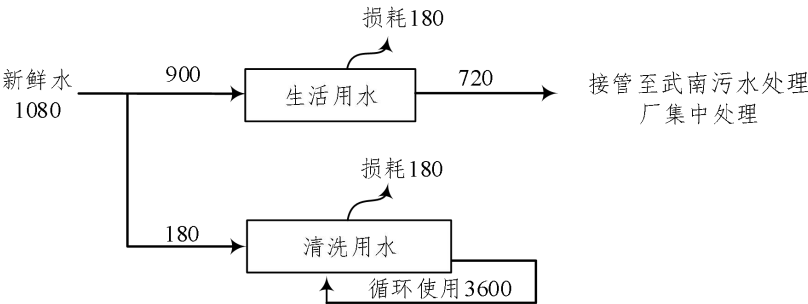
图 2-1 水平衡图
