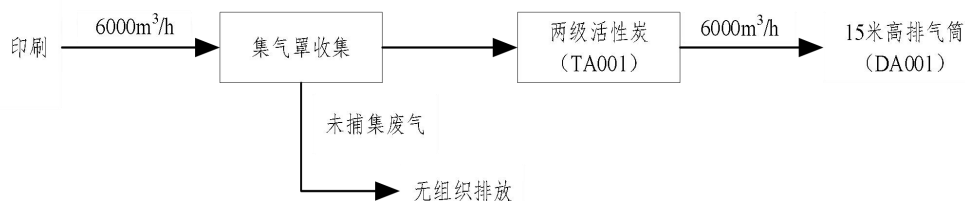
图 4-1 企业废气处理工艺图
