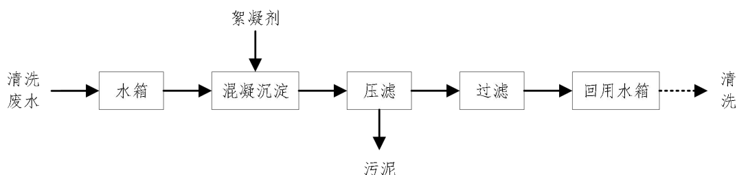
图 4-3 本项目废水处理工艺流程图
