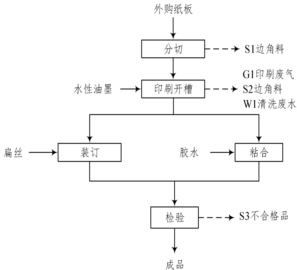
图2-3 工艺流程图
