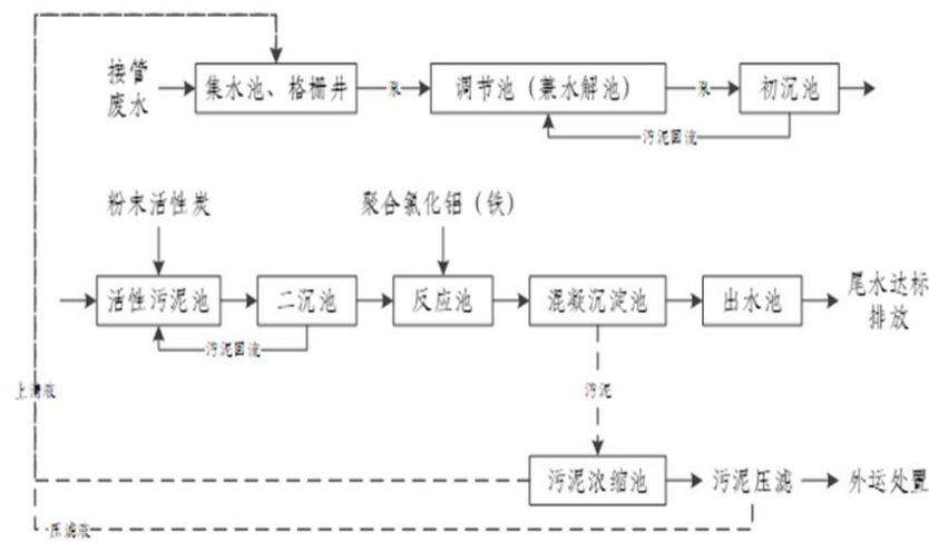
图4-2 武南污水处理厂污水处理工艺流程图
